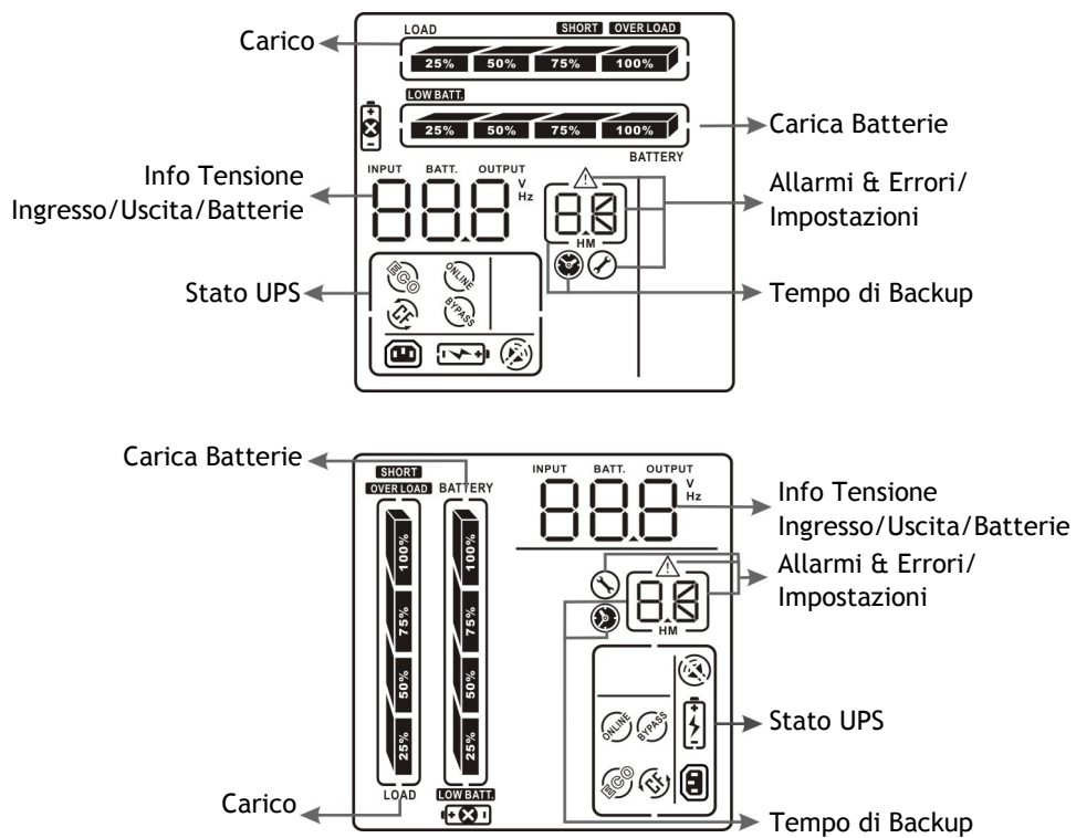
Figura 3 - Pannello LCD grafico
